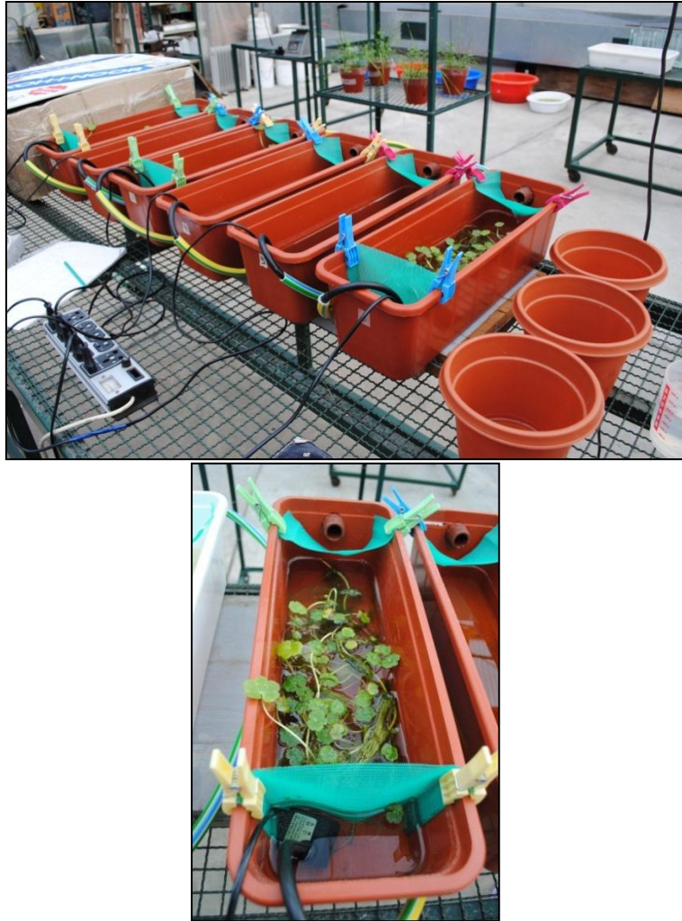
Figura 4.3. Disposición de los reactores utilizados en el bioensayo V (arriba) y detalle de uno de los reactores correspondiente al tratamiento Hr (abajo).
