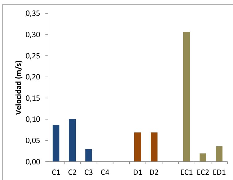
Figura 1.13. Velocidades superficiales de corriente (medias) en el centro del cauce en distintos sitios de los arroyos La Choza (C1 a C4) y Durazno (D1 y D2) y canales a cielo abierto (EC1, EC2 y ED1).
