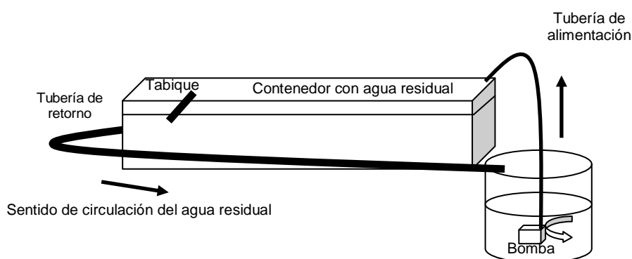
Figura 3.2. Esquema del sistema de recirculación del agua residual.
