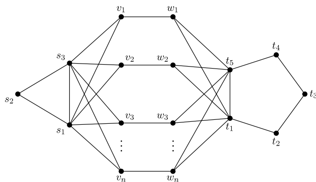
Fig. 6. Graphs T_n .
