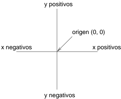
Coordenadas cartesianas
